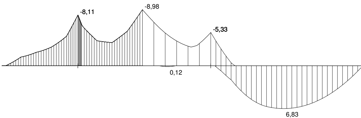
max.My,d - Grenzlinie für Holzträger [kNm]
