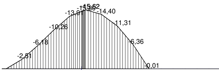
max.My,d - Grenzlinie für Verstärkung [kNm]
